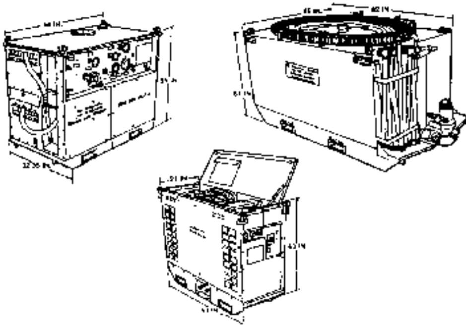
Figure A-III-1. M12A1 PDDA.
